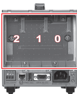
Задняя сторона GX10
