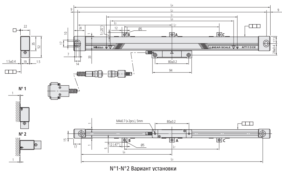
N°1-N°2 Вариант установки
